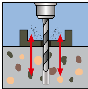
2. Remove dust
